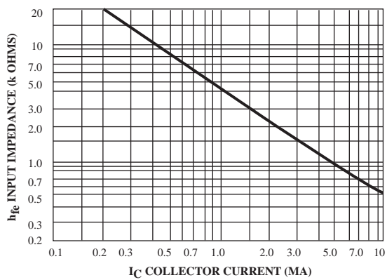
FIG.11 Input Impedance
