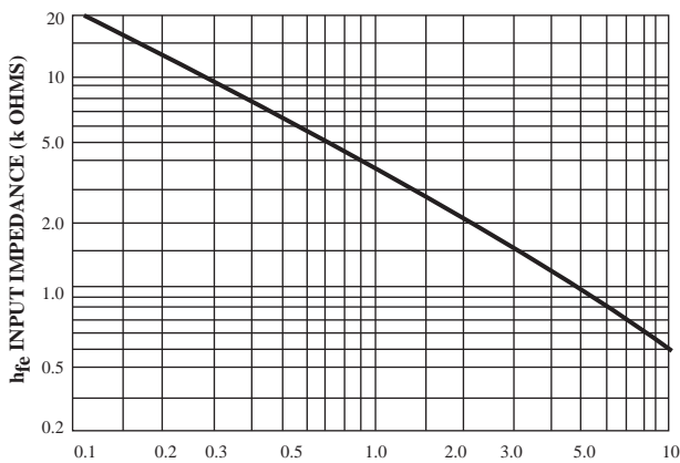
FIG.13 Input Impedance
